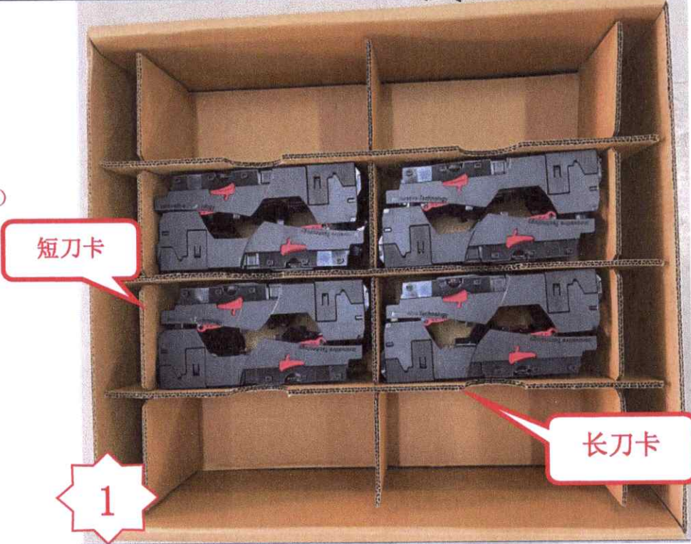
图一, 将 PA2613 按照每格 2pcs, 每层 8 格, 每箱 2 层的方式包装, 同时在底层, 中层, 顶层各放一块隔板, 共 3 块隔板。
